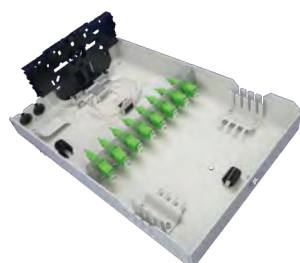
Boîtier de couplage secondaire 1:8 IB1443
